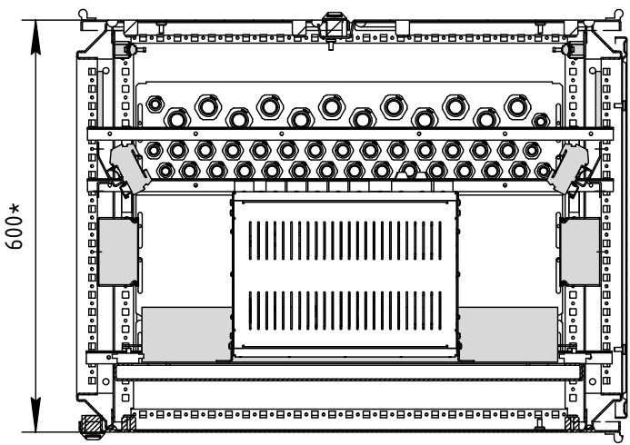
A-A
