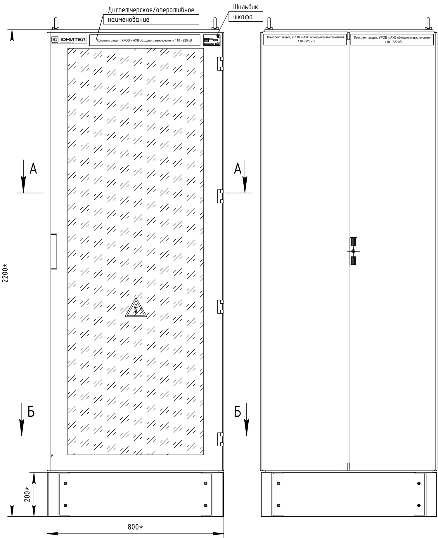
Вид сзади
